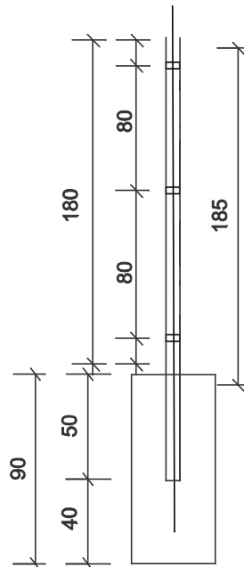
PRZEKRÓJ I-I
