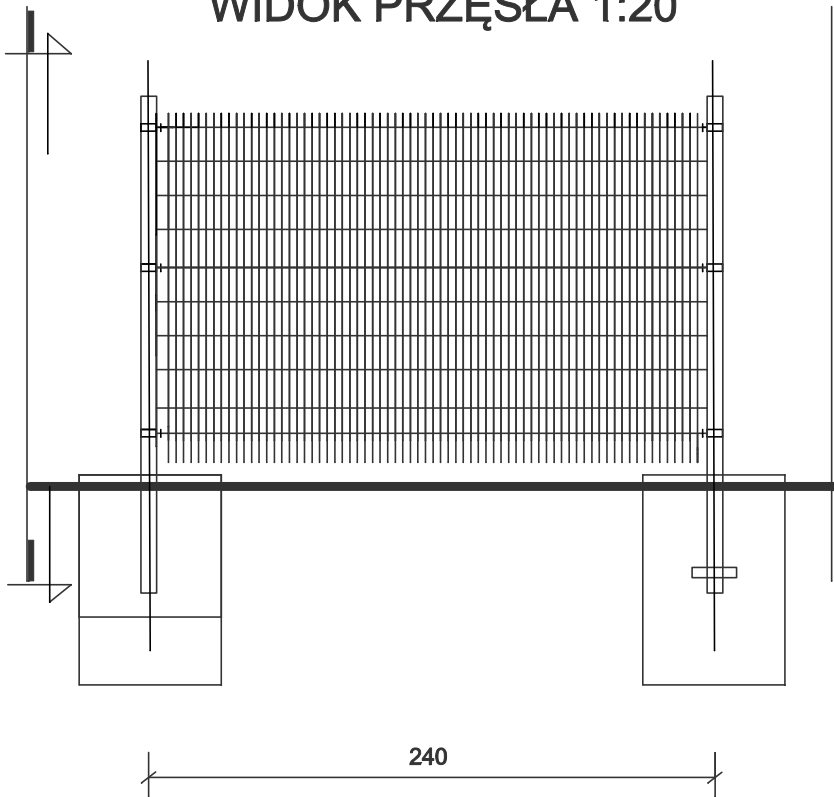
WIDOK PRZĘSŁA 1:20
